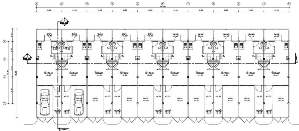
แปลนพื้นที่ล่าง 1:125
