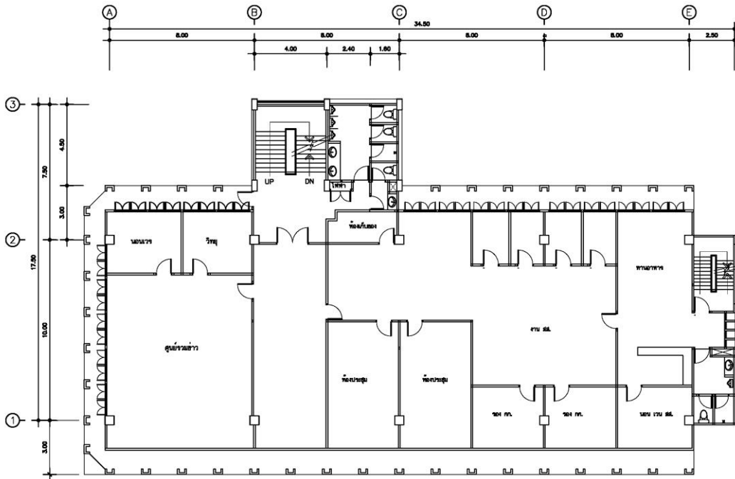
แปลนพื้นที่ 4
