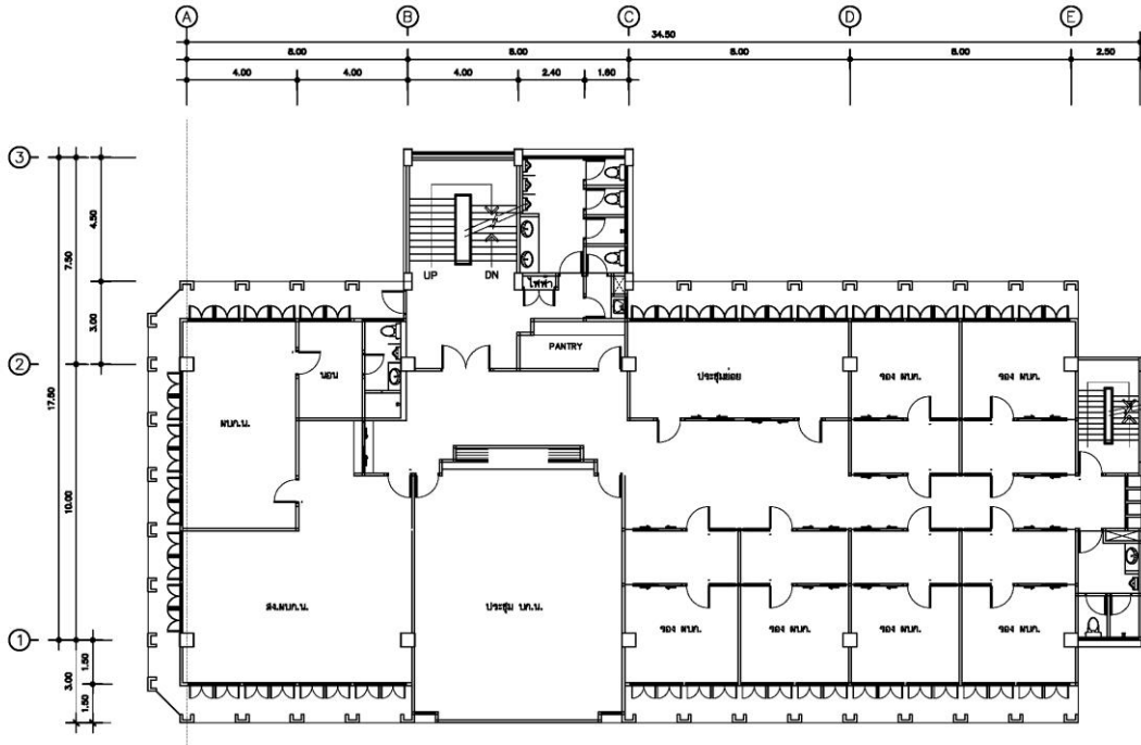
แปลนพื้นที่ 3
