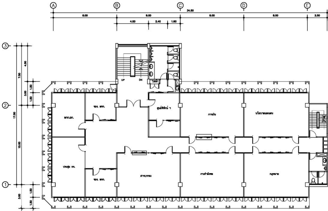
แปลนพื้นที่ ชั้นที่ 2
