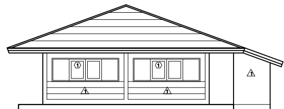
รูปด้าน C 1 : 100
