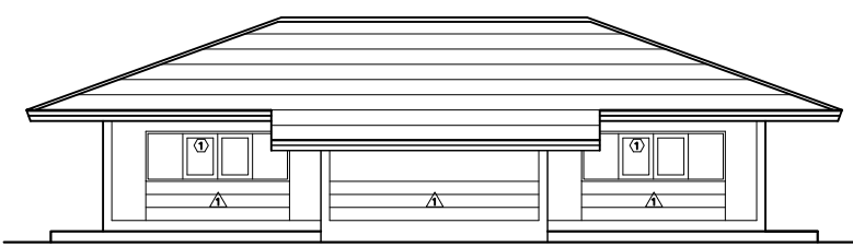
รูปด้าน D 1 : 100
