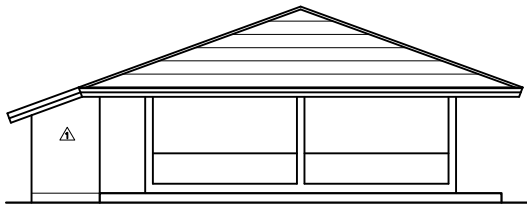
รูปด้าน B 1 : 100
