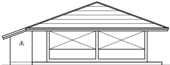
รูปด้าน B 1 : 100
