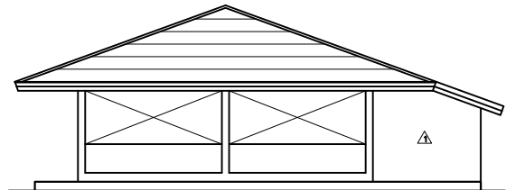
รูปด้าน D 1 : 100
