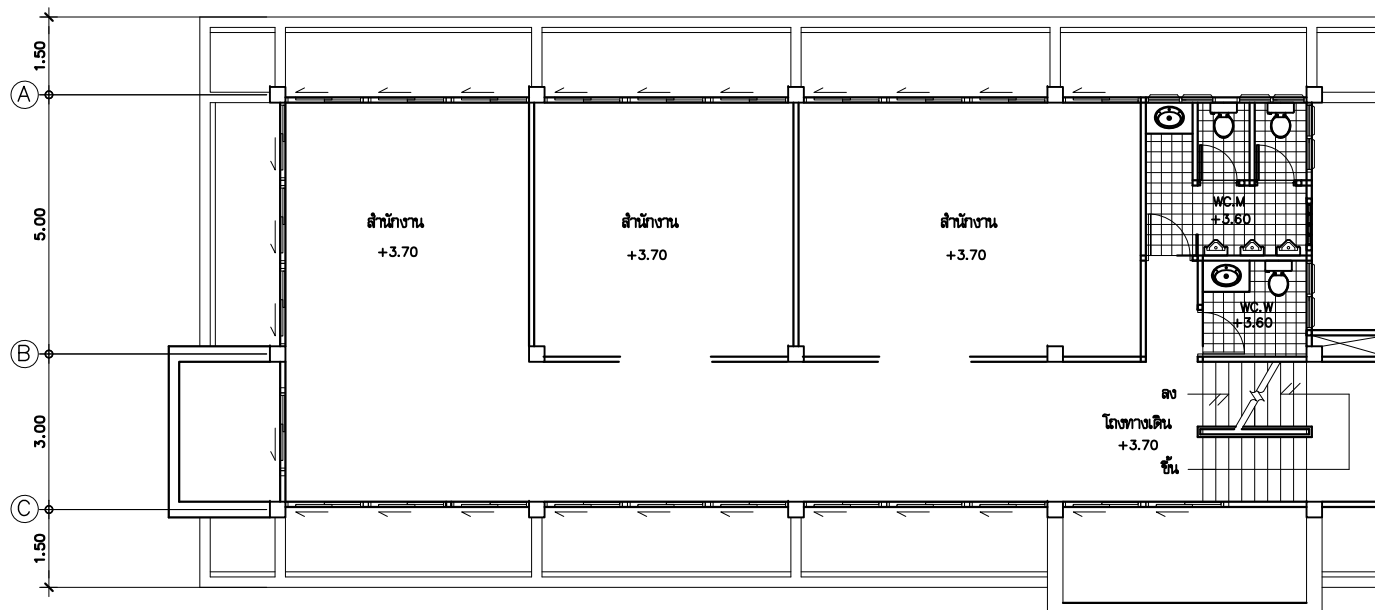
แปลนชั้นที่ 2
