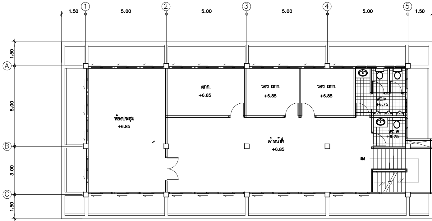
แปลนชั้นที่ 3
