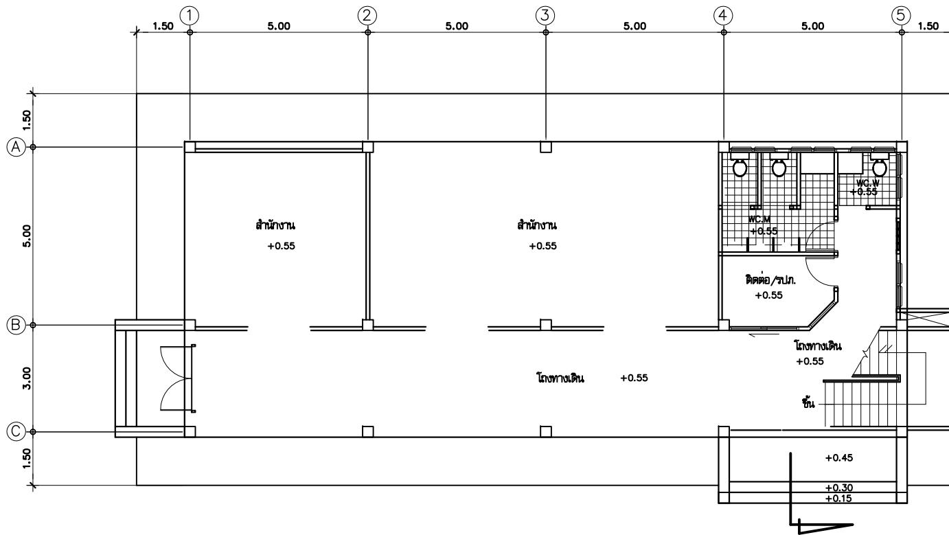
แปลนชั้นที่ 1
