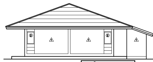
รูปด้าน C 1 : 100
