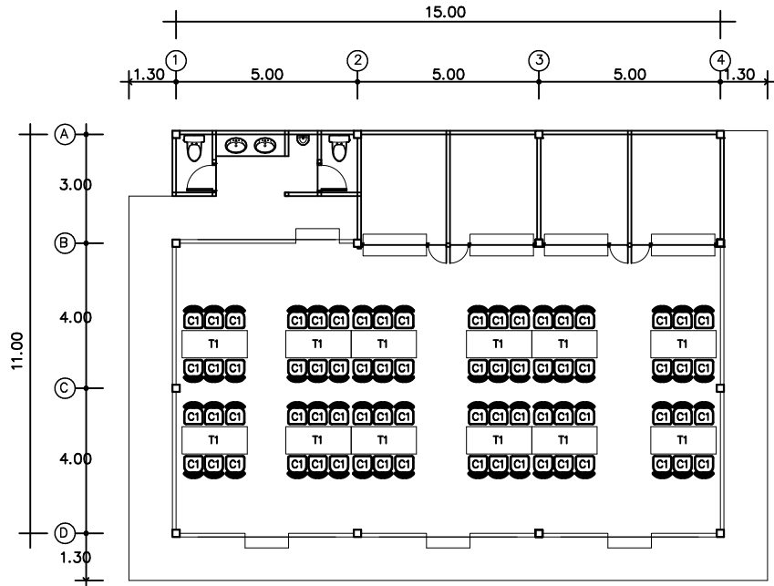
ผังคู่มือ 1 : 100
