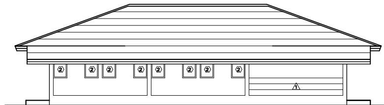
รูปด้าน D 1 : 100
